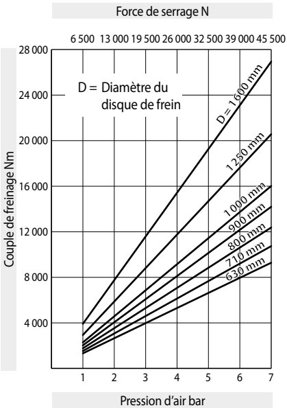
Pince de frein DU 060 PFM - 680
