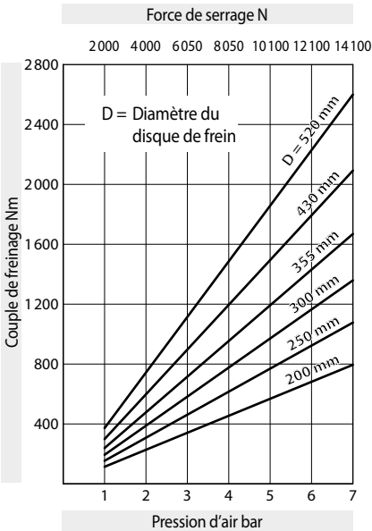
Pince de frein DH 030 PFM - 655
