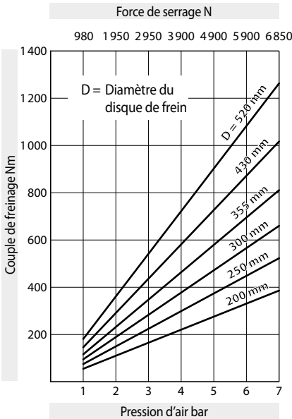
Pince de frein DH 025 PFM - 635
