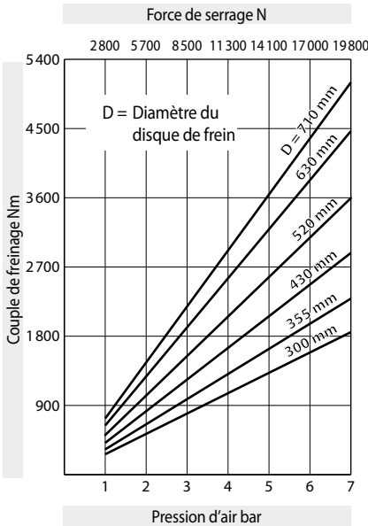
Pince de frein DV 035 PFM - 660
