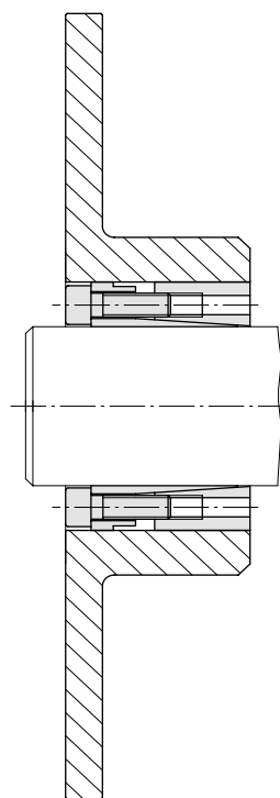
Assembleur expansible RLK 130 avec disque de frein forme B
