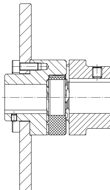
Accouplements à doigts REK ... DCS avec disque de frein Forme F
