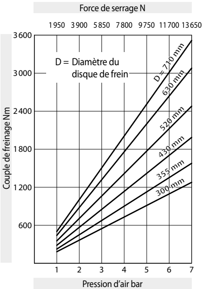
Pince de frein DV 035 PFM - 655
