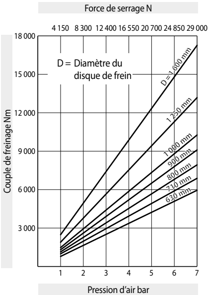
Pince de frein DU 060 PFM - 660
