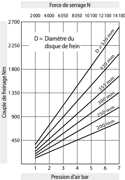
Pince de frein DH 025 PFM - 655
